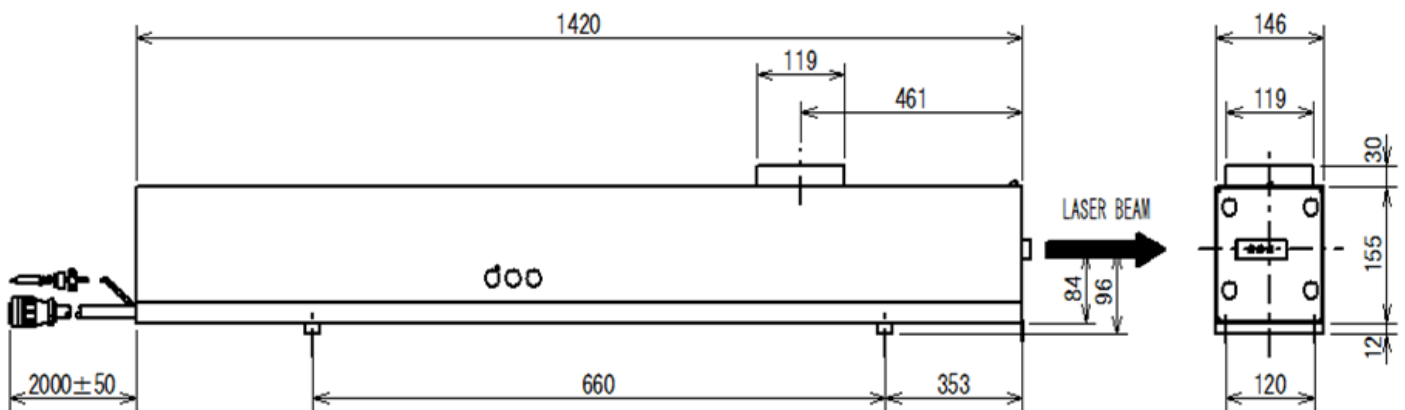
外形図 (mm) IK-G
