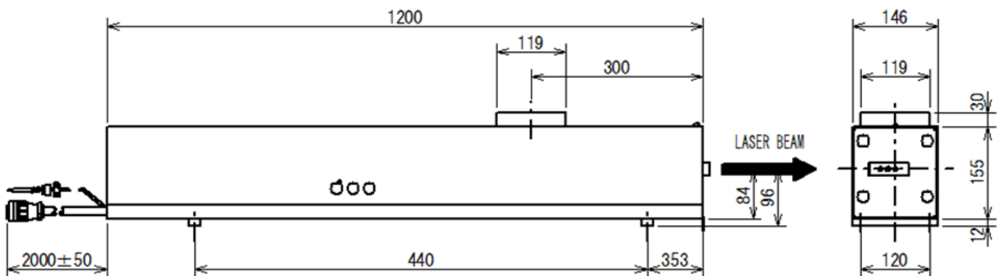
外形図 (mm) IK-F
