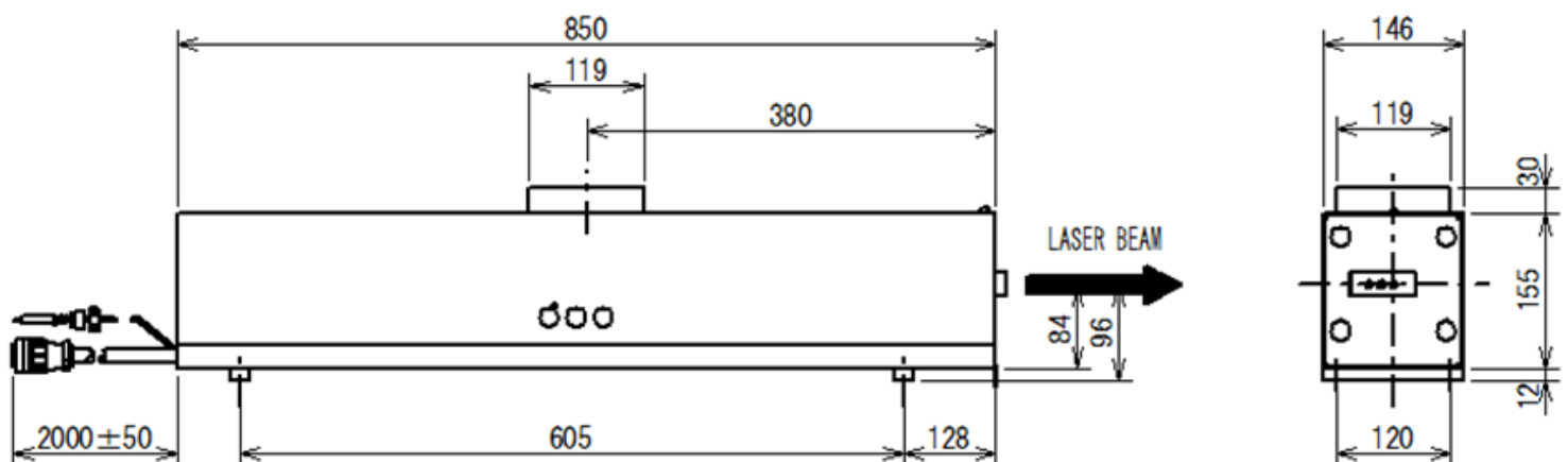
外形図 (mm) IK-D
