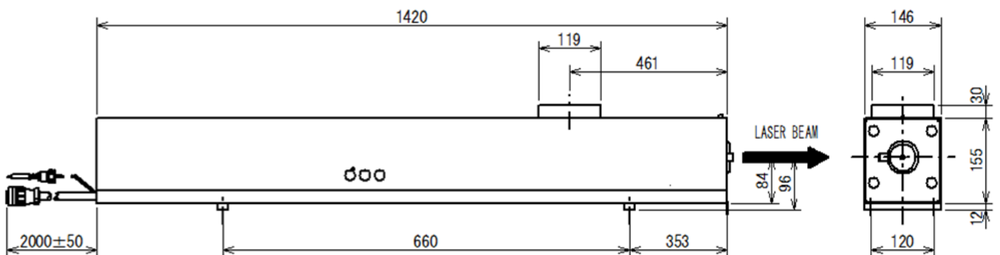
外形図 (mm) IK-G
