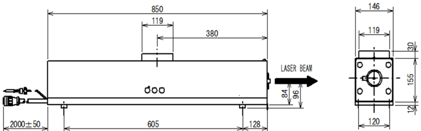
外形図 (mm) IK-D
