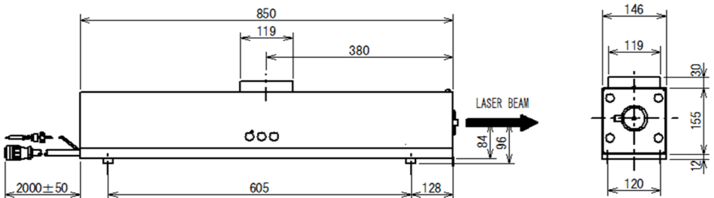
外形図 (mm) IK-D
